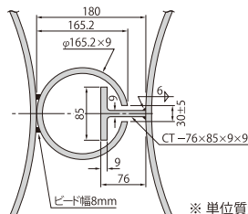
P-T型 (φ165.2×9, CT-76×85×9×9)
