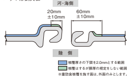
ハット形鋼矢板
