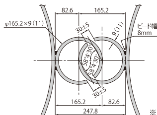
P—P型 (φ165.2×9 (11))
