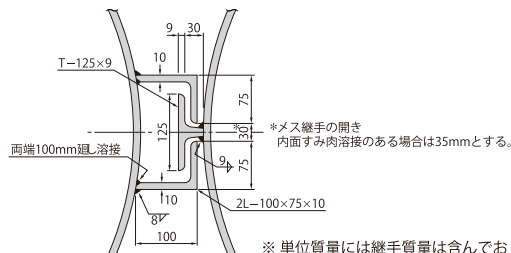
L-T型 (L-100×75×10, T-125×9)
