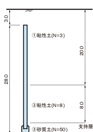
地盤柱状図
