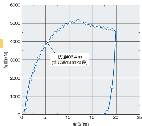
管内リングと球根との付着試験結果
