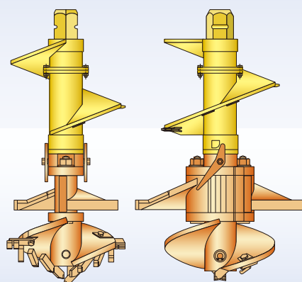
Bタイプビット 概要 (根固め倍率1.25または1.5倍)
