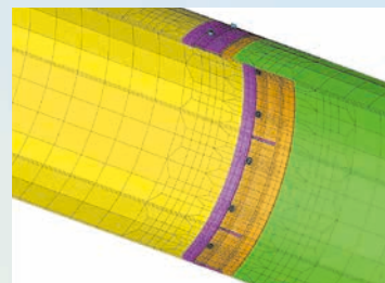
要素分割図 (継手部拡大)
