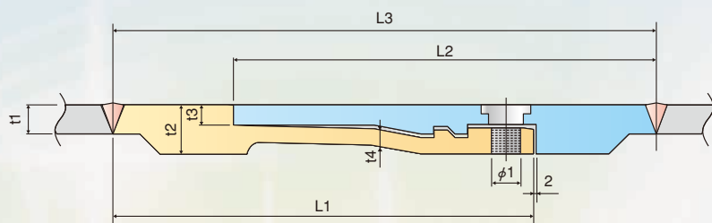
■カシーン標準寸法表 (SKK490)
