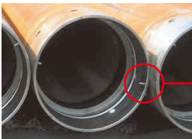
芯合わせ用ボルト
