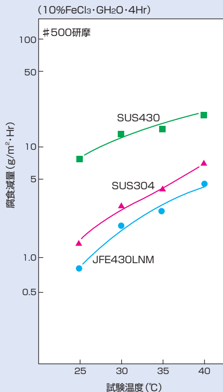
図-1. JFE430LNMの孔食試験結果 (腐食減量がいさいほど点錆抵抗が大きい)
