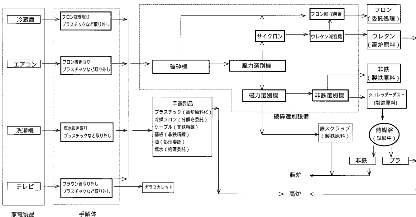
図1 処理フロー
