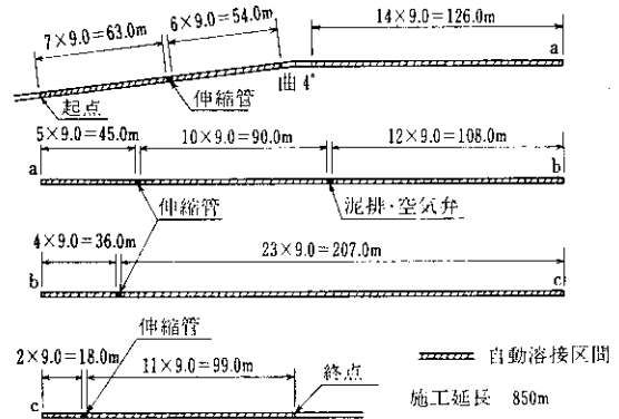
図1 管割図
