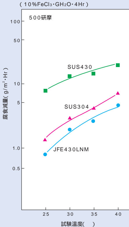
図-1 .JFE430LNMの孔食試験結果 (腐食減量が小さいほど点錆抵抗が大きい)
