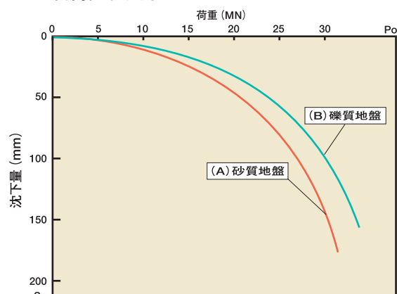
杭頭荷重 P_0 ～杭頭沈下量 S_0 曲線
