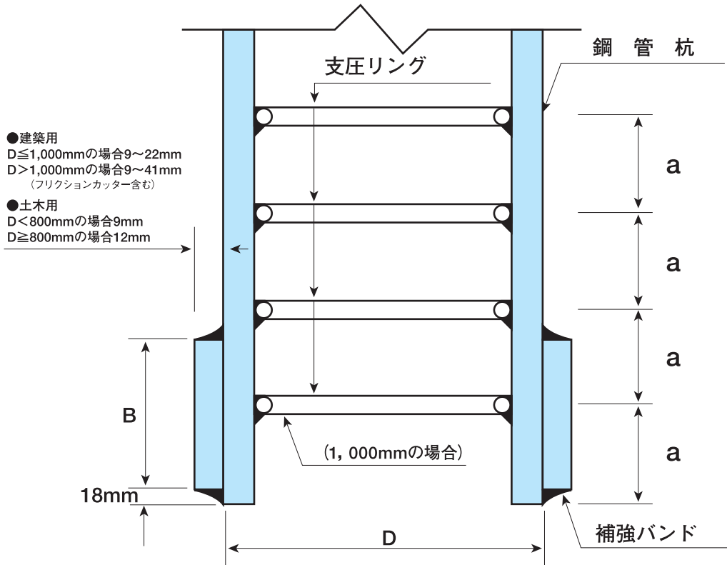
杭先端支圧リング、杭先端補強バンド標準仕様
