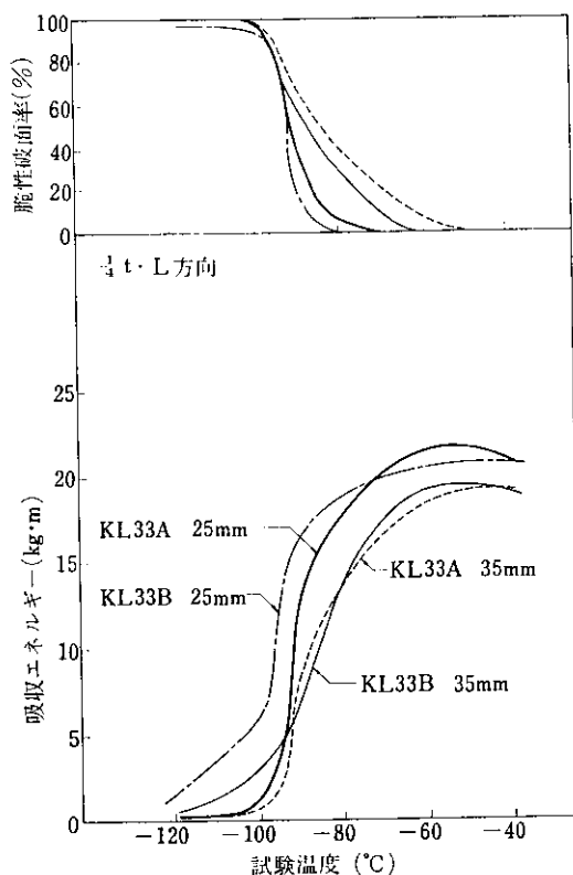
図5 KL33A, KL33B の 2 mmV ノッチシャルピー衝撃試験結果
