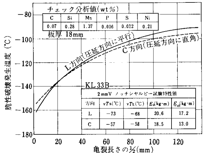
図 10 無限板の場合の亀裂長さとの関係 ( \sigma = \sigma_y/2 )
