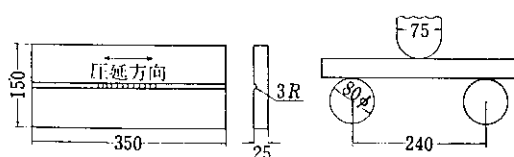
図 15 溶接ビード曲げ試験片および治具形状
